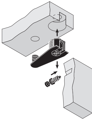
Outtrigger - 16 mm (5/8")
